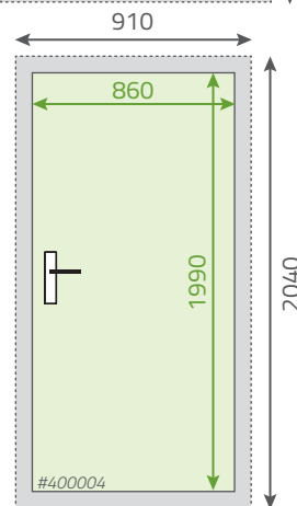
③ Kabinentür 2
